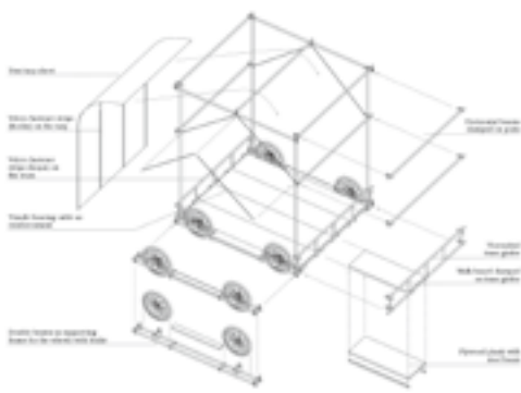
构造分解图
