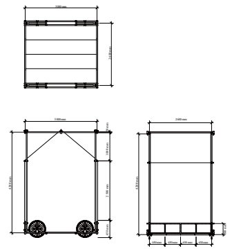
技术图
