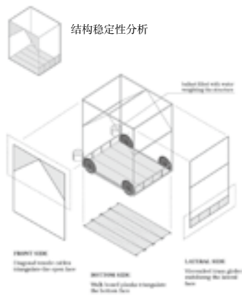
结构示意图
